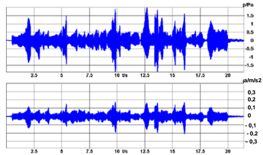
Abbildung 1: oben: zeitliche Sequenz einer Luftschallaufnahme von einem Orgelstück; unten: zeitliche Sequenz der Schwingungsaufnahme.
